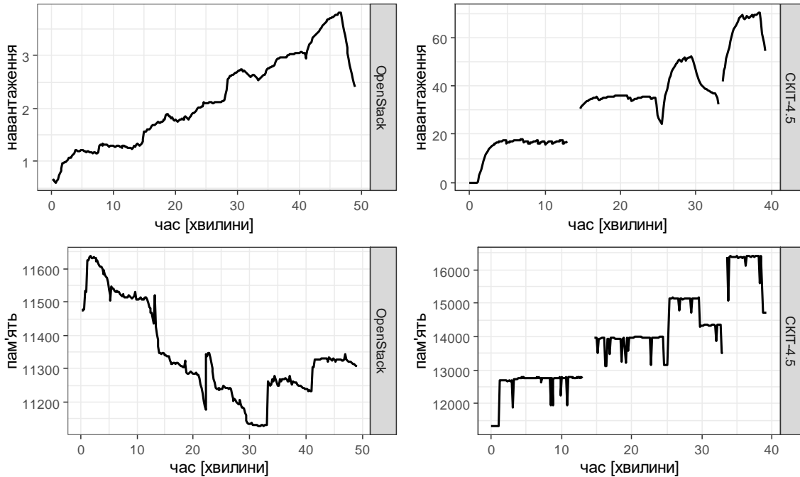
РИС. 3. Порівняння навантаження та використання оперативної пам'яті для серверів OpenStack та СКІТ-4.5 при послідовному виконанні 4-х крос-валідацій із збільшенням кількості паралельних процесів з 1 до 4
