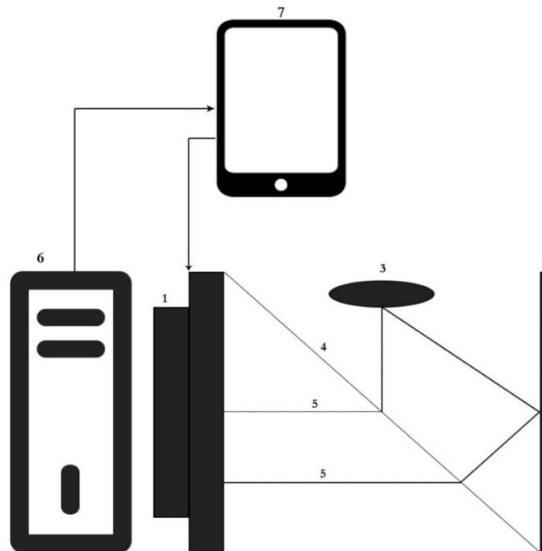
РИСУНОК. Схема функціонування голографічної 3D-вітрини
