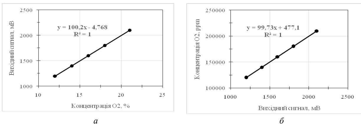
РИС. 8. Залежності газоаналізатора для кисню: a – калібрувальна, б – градувальна
